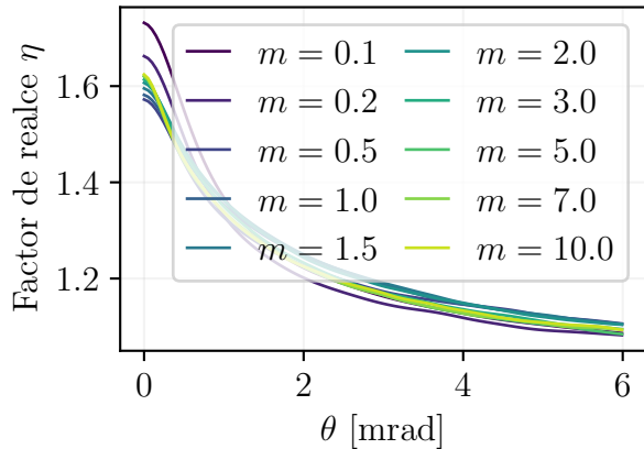
(a) cono completo (escala de \ell_{\text{bot}}^* )
