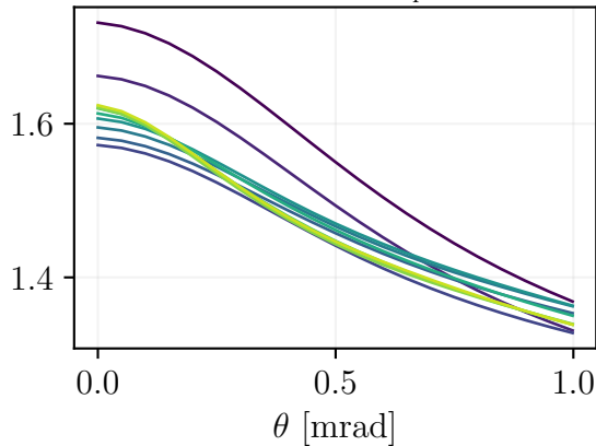
(b) ápice (escala de \ell_{\text{top}}^* )
