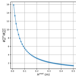
Concentration de flux vs. hauteur de la couche métal (cf. TD)
