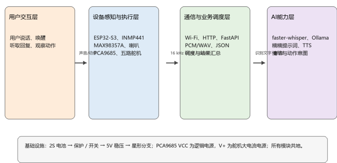
图 2-1 毛绒陪伴机器人四层总体架构（初版）
