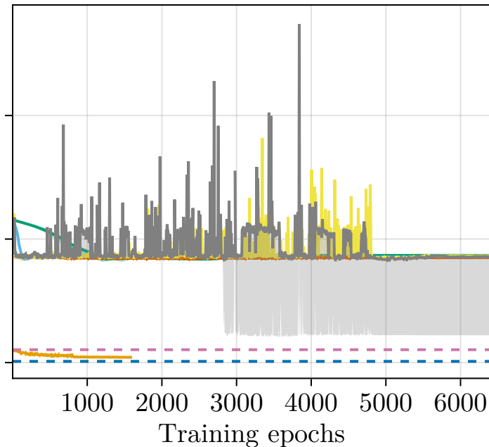
MLP
