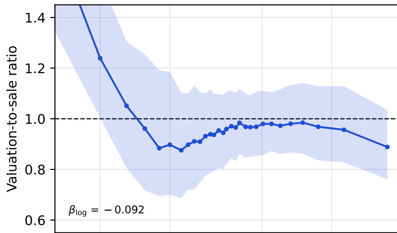
Held-out Linear
