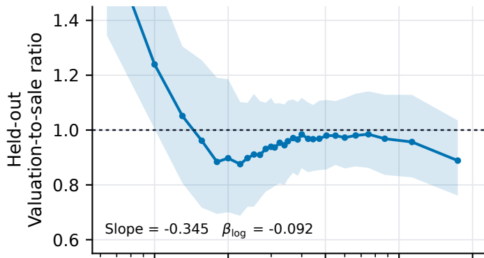
Linear regression
