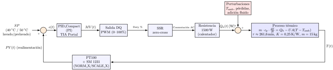
Figura 9: Diagrama de bloques del sistema térmico.
