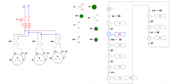
Figura 10: Etapa 2: Calentamiento del agua mediante resistencia de inmersión.
