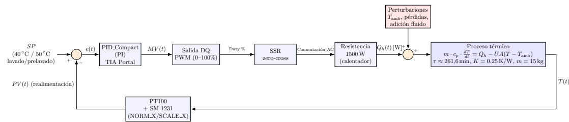
Figura 8: Diagrama de bloques del sistema térmico.
