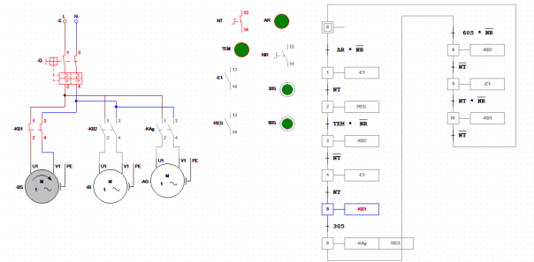
Figura 14: Etapa 5: Dosificación del jabón.
