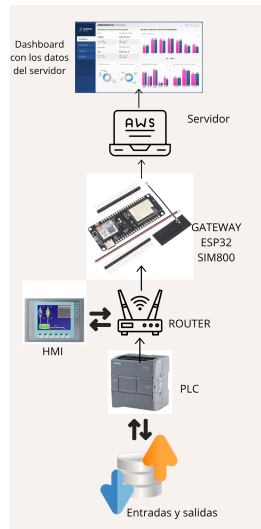
Figura 24: Arquitectura de comunicaciones propuesta.
