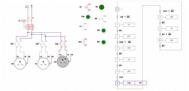
Figura 14: Etapa 6: Agitación y calentamiento de la mezcla de agua y sustancia de limpieza.
