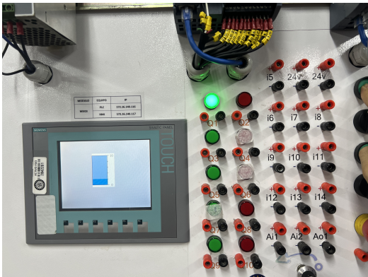
Figura 27: Accionamiento e interfaz del panel HMI.
