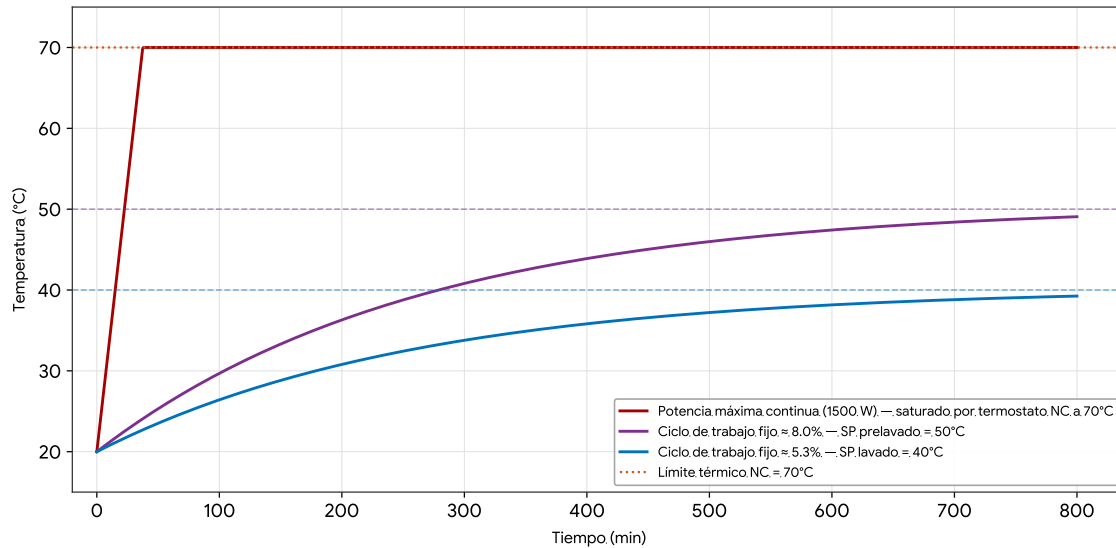
Figura 25: Respuesta preliminar del modelo en lazo abierto.
