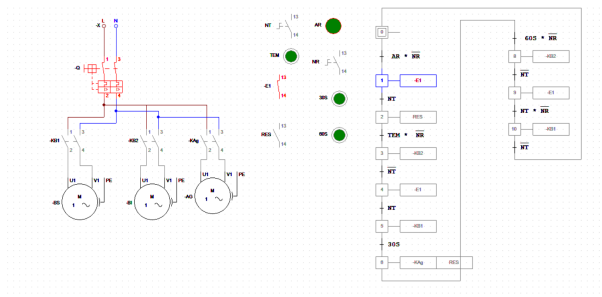
Figura 9: Etapa 1: Llenado de la cabina de operaciones.
