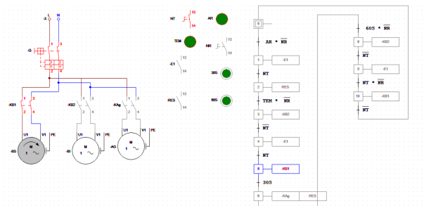
Figura 13: Etapa 5: Dosificación del jabón.
