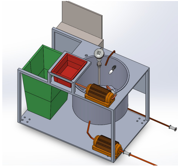
Figura 22: Vista isométrica lateral del sistema CIP. Destaca la disposición de la bomba de recirculación en la parte inferior y las líneas de tubería de impulsión y retorno.
