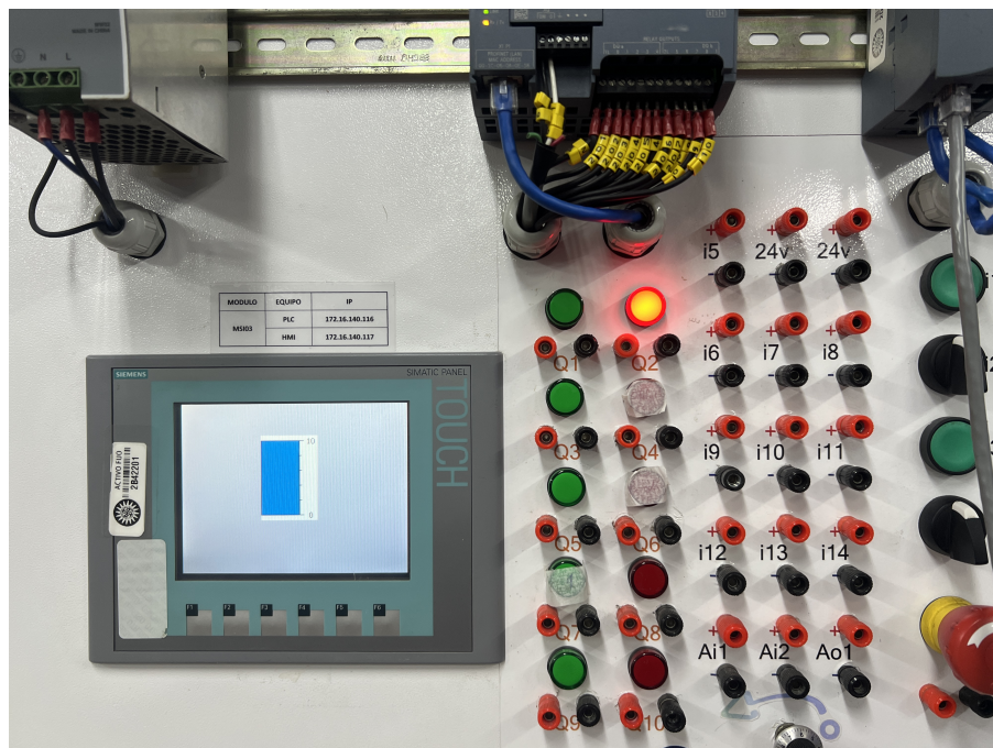
Figura 29: Simulación de la condición de tanque lleno.
