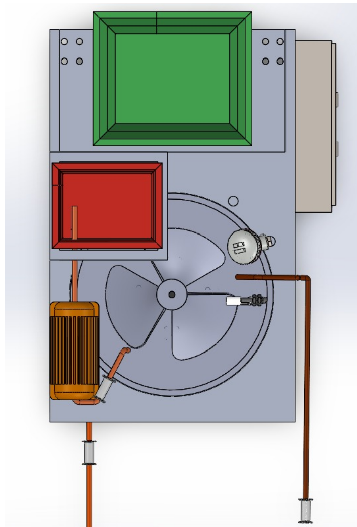
Figura 20: Vista superior del sistema CIP. Se observa el tanque principal con el agitador, el sensor de temperatura, la sonda lateral y el tanque de químicos (rojo).
