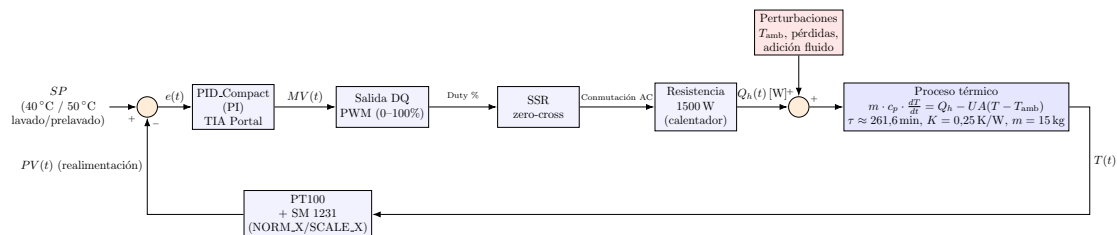
Figura 24: Diagrama de bloques del sistema térmico.
