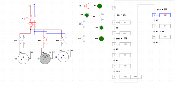
Figura 15: Etapa 7: circulación de la solución de limpieza en la tubería.
