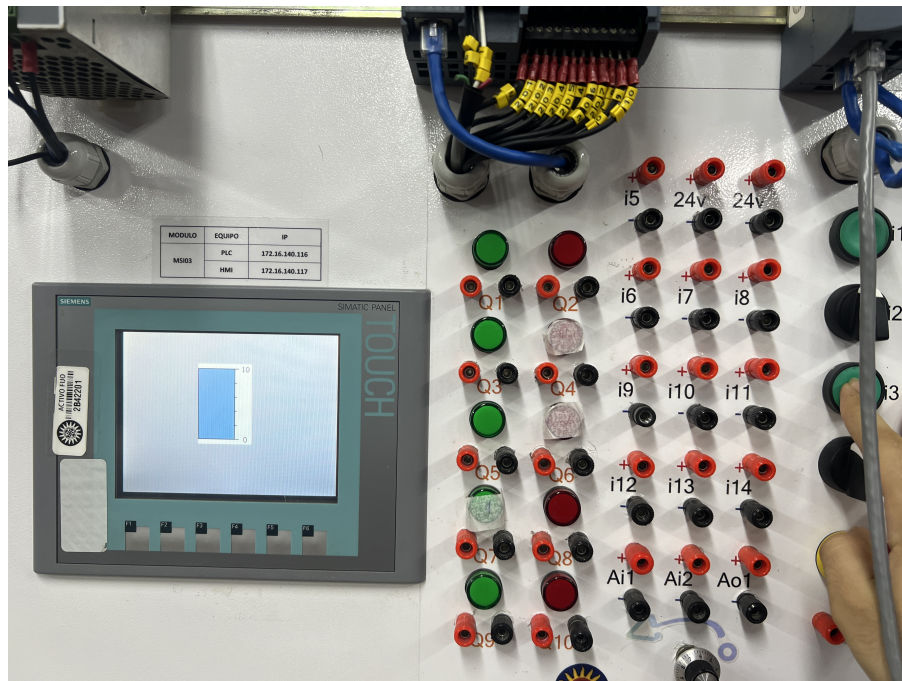
Figura 28: Reinicio y reseteo de estados del sistema.
