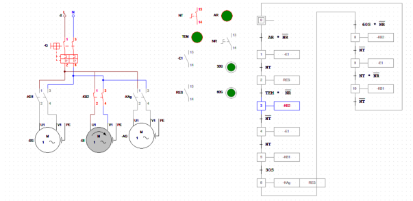
Figura 11: Etapa 3: Bomba de drenado de la cabina de operaciones.
