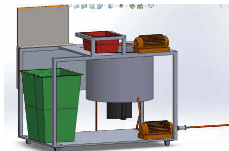
Figura 21: Vista isométrica general del sistema CIP. Se aprecia la estructura con ruedas, el tanque principal, el motor del agitador, la bomba inferior y los contenedores de químicos (rojo) y auxiliar (verde).
