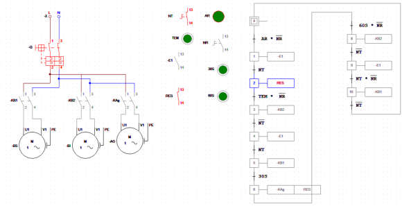
Figura 10: Etapa 2: Calentamiento del agua mediante resistencia de inmersión.
