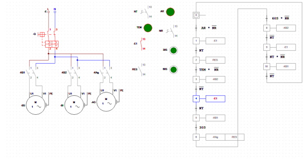
Figura 12: Etapa 4: Rellenado de la cabina de operaciones.
