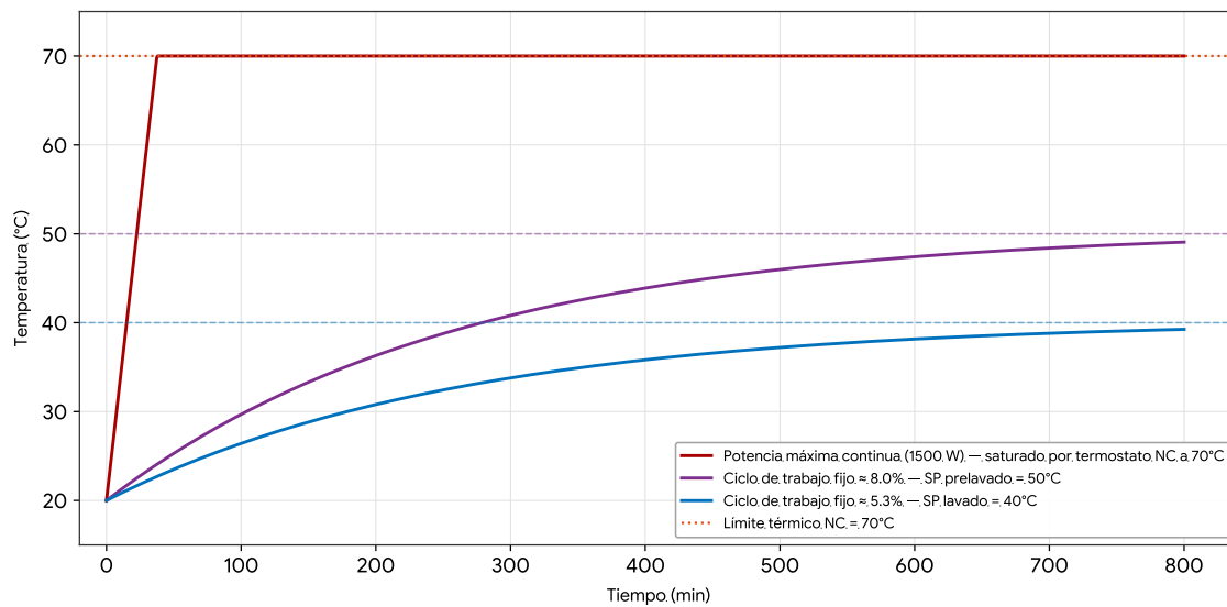
Figura 8: Respuesta preliminar del modelo en lazo abierto.
