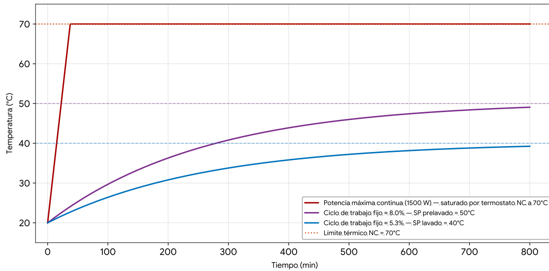
Figura 13: Respuesta preliminar del modelo en lazo abierto.
