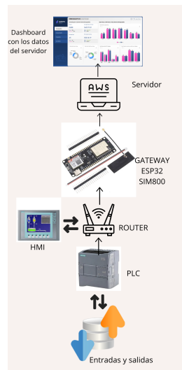
Figura 14: Arquitectura de comunicaciones propuesta.
