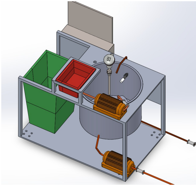
Figura 6: CAD general del sistema CIP.
