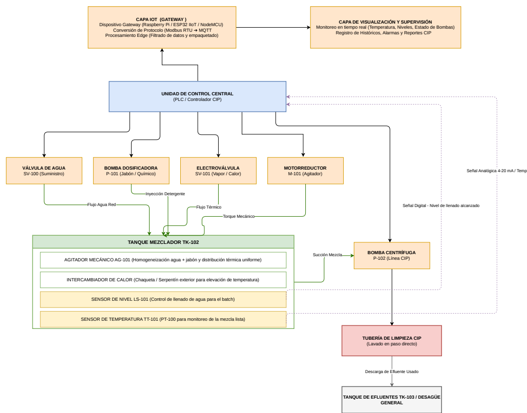
Figura 4: Arquitectura funcional del sistema.
