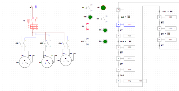
Figura 10: Etapa 1: Llenado de la cabina de operaciones.
