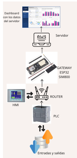
Figura 25: Arquitectura de comunicaciones propuesta.
