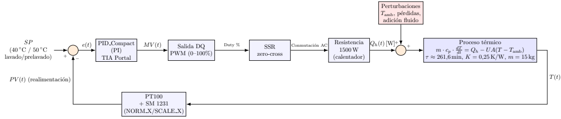
Figura 23: Diagrama de bloques del sistema térmico.
