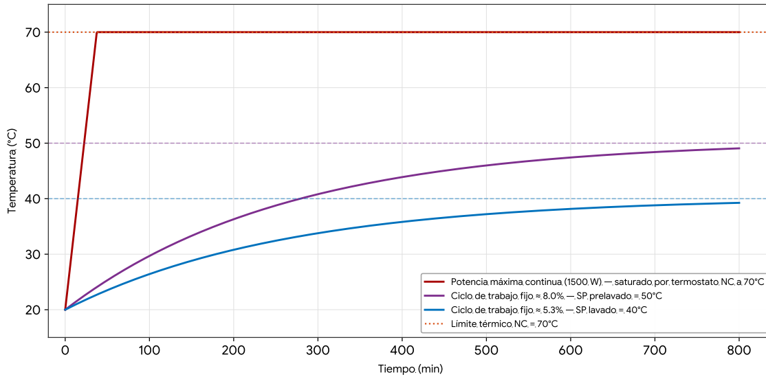
Figura 24: Respuesta preliminar del modelo en lazo abierto.
