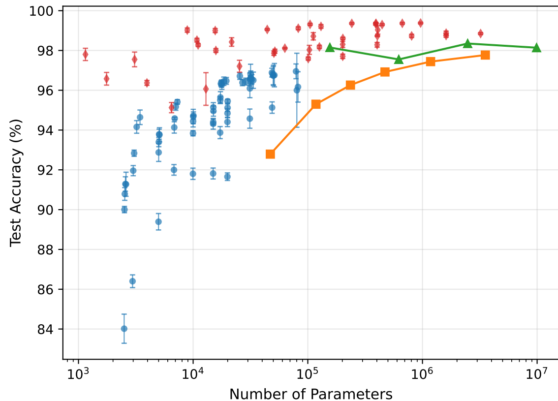
MNIST
