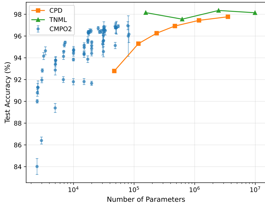
MNIST
