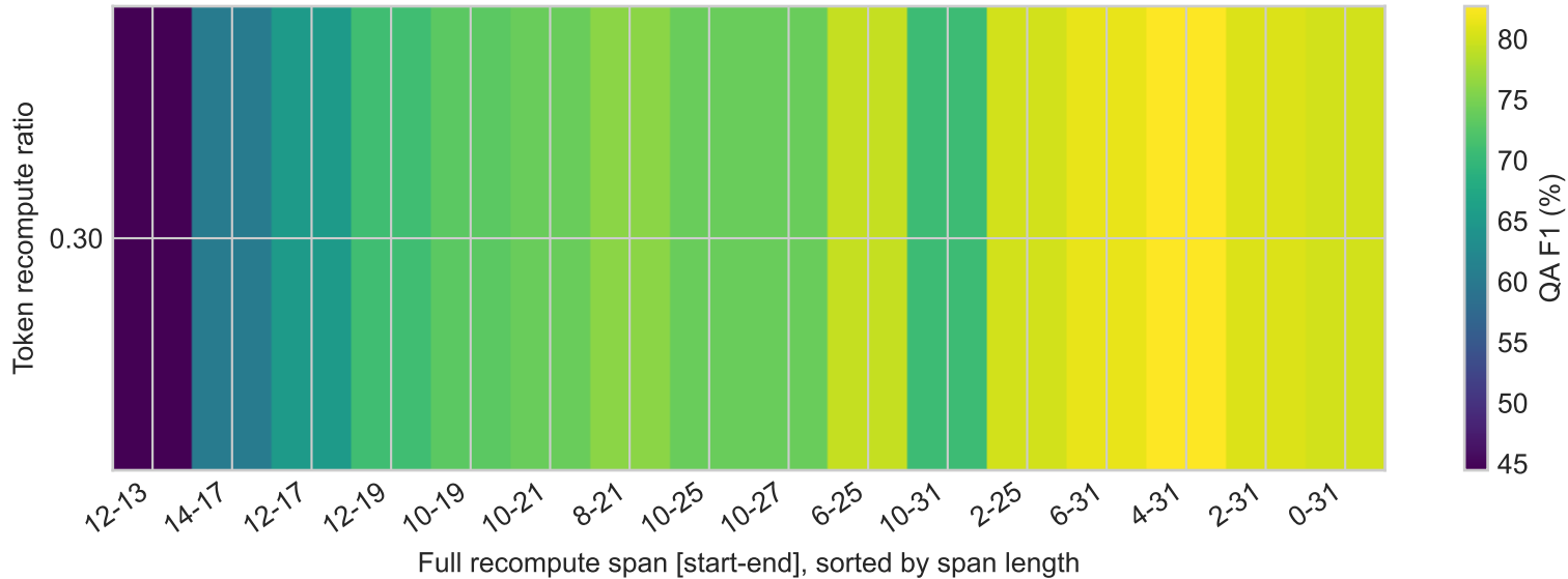
DroidBlend F1 heatmap: hotpotqa_50
