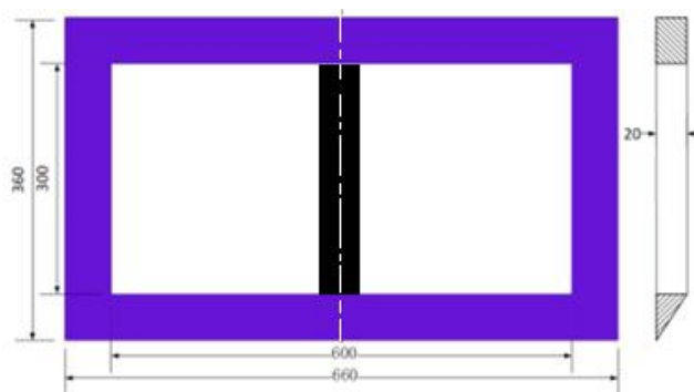
图7 安全区围栏示意图
