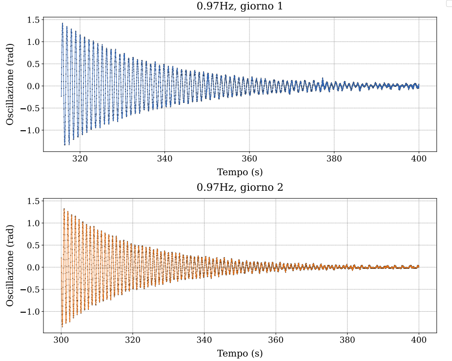
Figura 4: Confronto del moto smorzato (con correzione di offset già applicata): sopra la prima giornata, sotto la seconda
