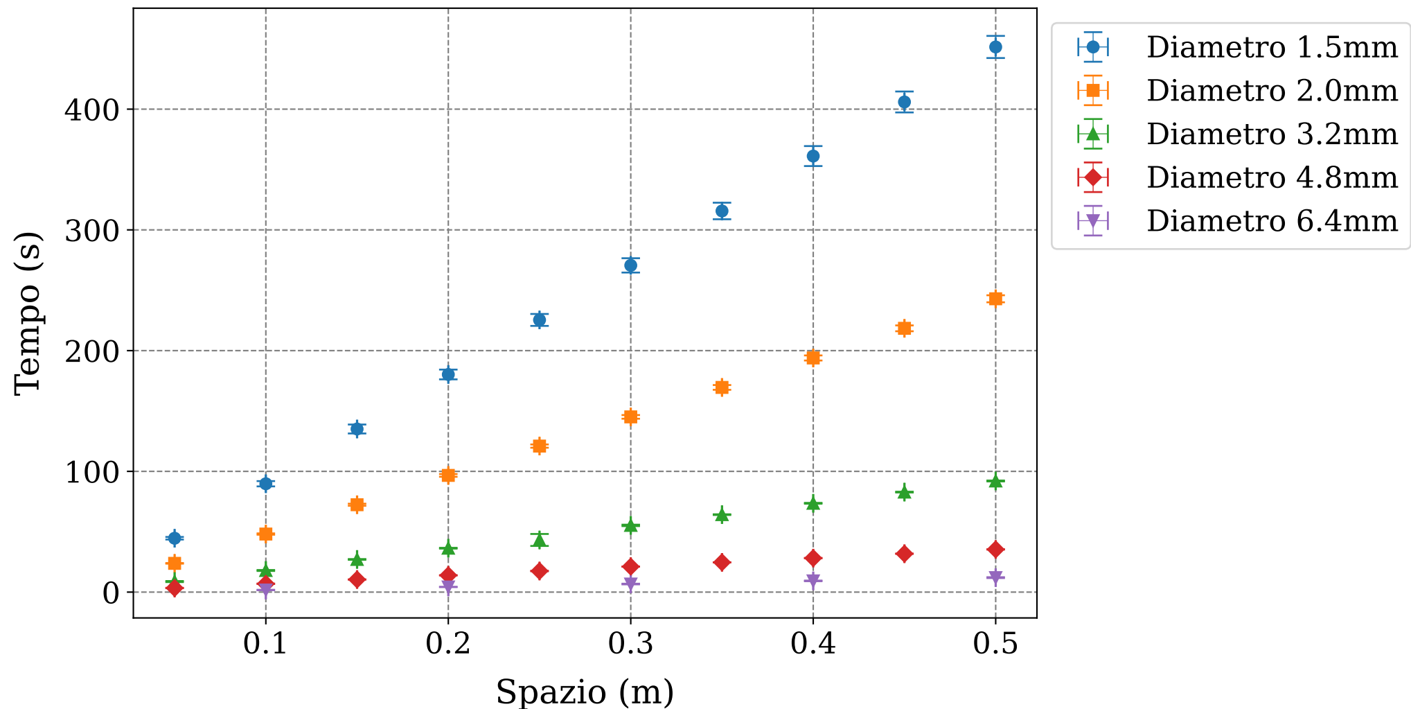
Sapone: Confronto andamento dei tempi di caduta
