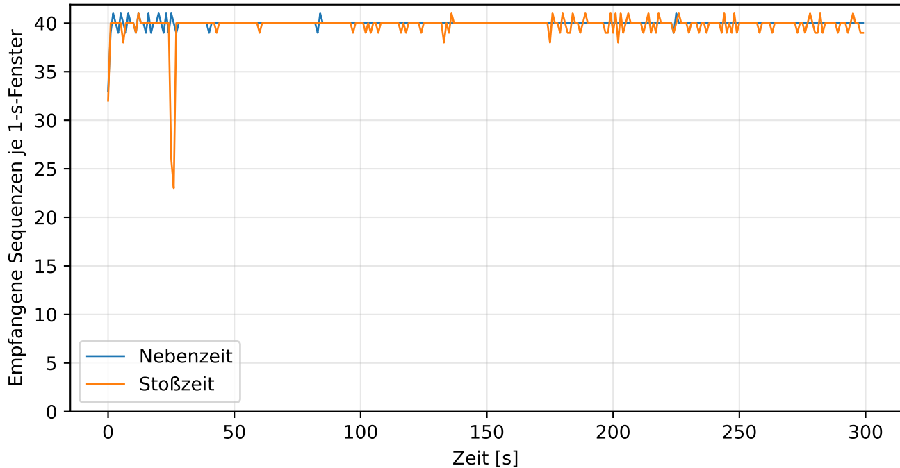
Empfangene Sequenzen über die Zeit (Störfestigkeit)
