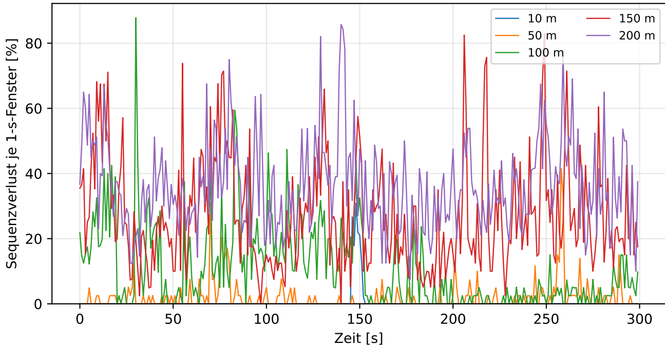
Reichweite (ohne Sichtverbindung): zeitlicher Verlauf des Sequenzverlusts
