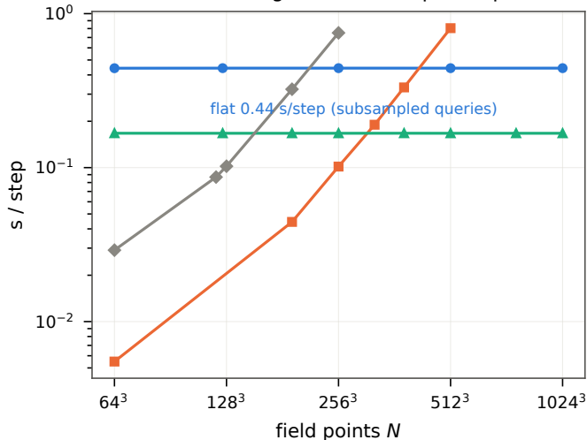
(d) training — wall-clock per step
