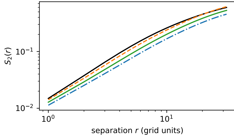
Longitudinal structure function
