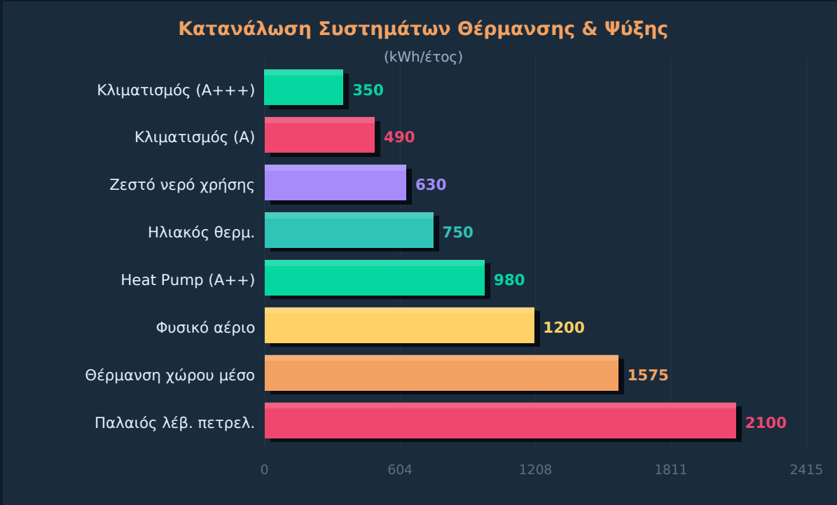
Σχήμα 2: Σύγκριση ετήσιας κατανάλωσης συστημάτων θέρμανσης & ψύξης (IEA 2024)
