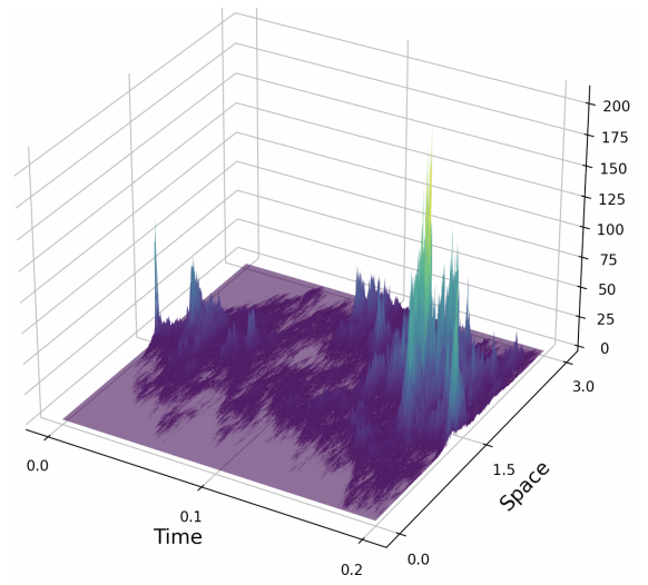
(d) \lambda = 2
