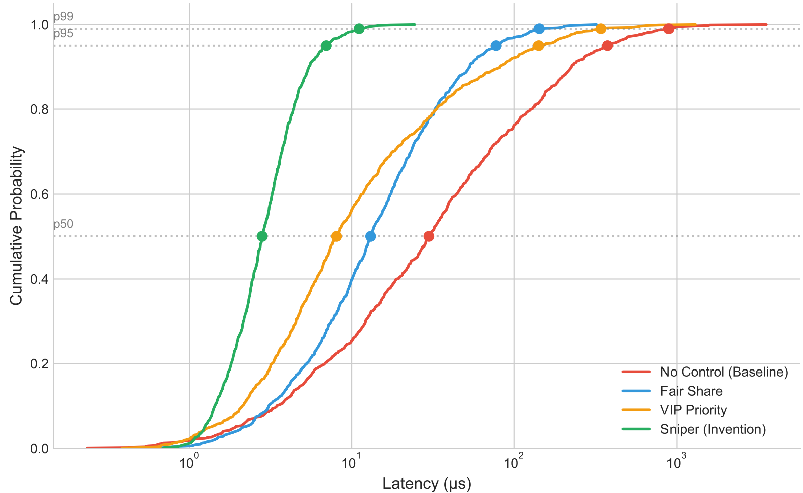
Good Tenant Latency CDF
