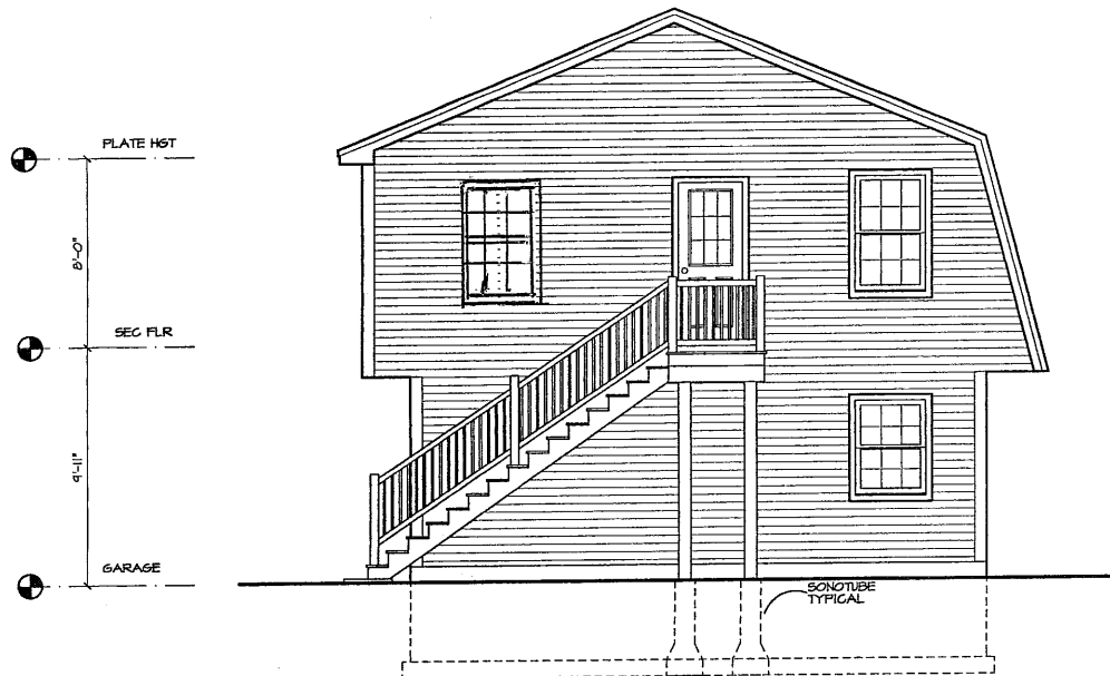
1 LEFT SIDE ELEVATION A3 SCALE: 1/4" = 1'-0"
