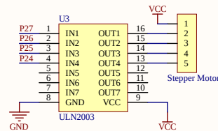
步进电机
