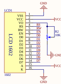
液晶模块
