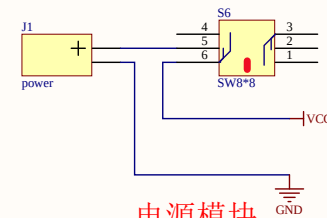
电源模块
