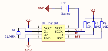
时钟模块
