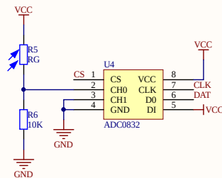
光敏模块
