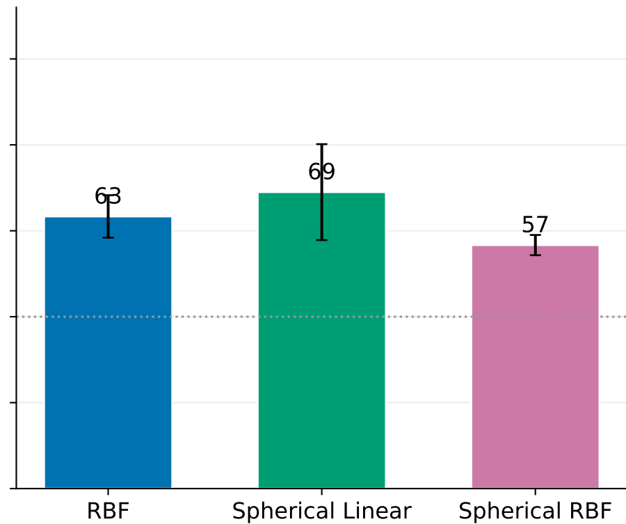
Erdos100
