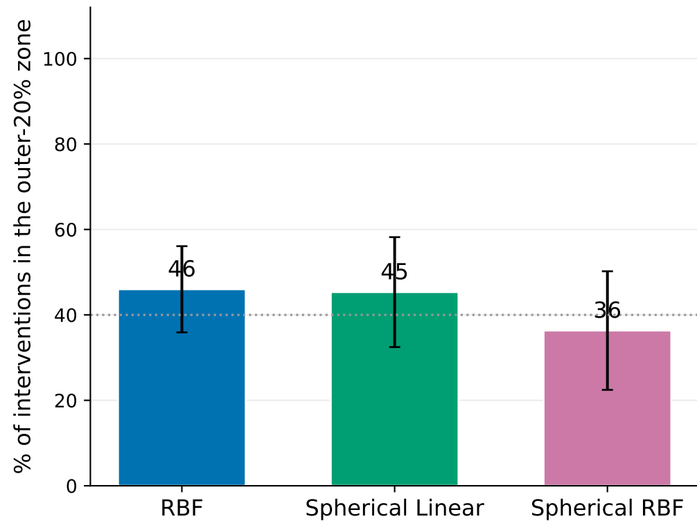
Erdos50
