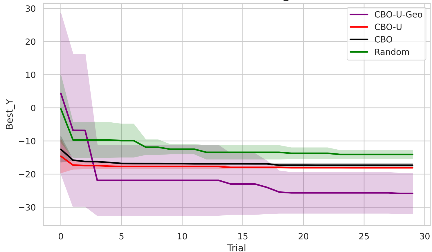
Erdos50 (linear) - Best_Y
