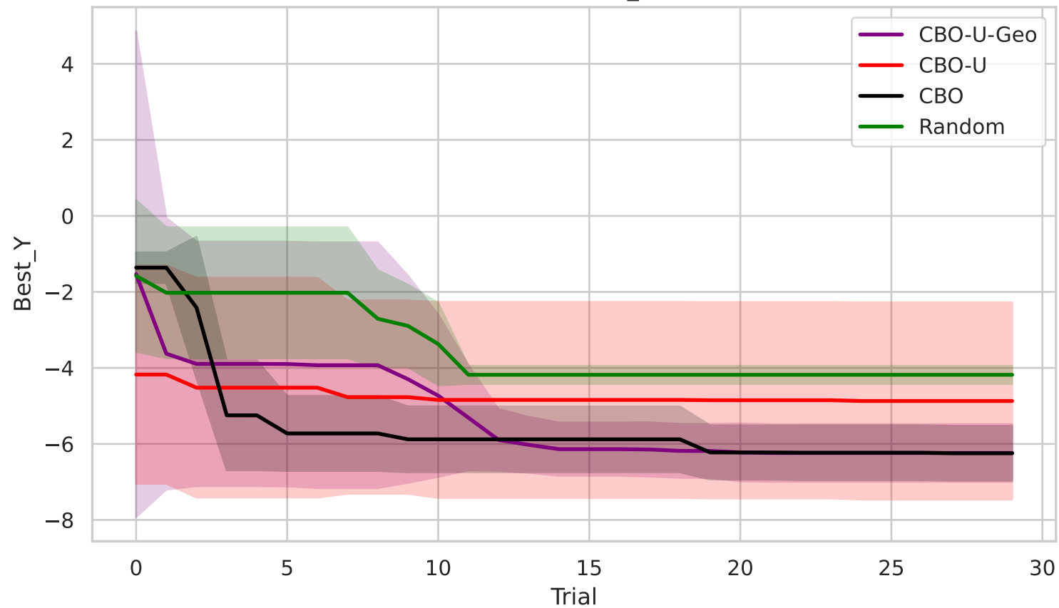
K562 - Best_Y
