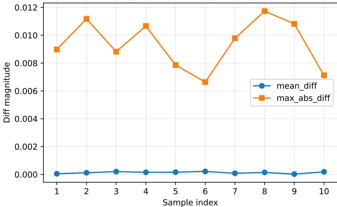
Noisy CF robustness per sample
