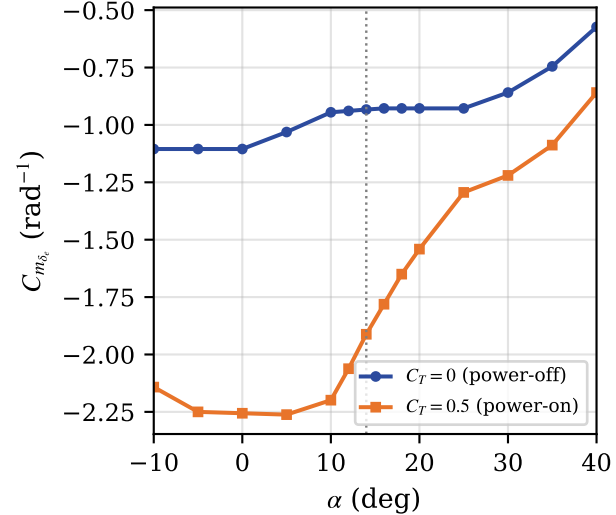
(d) Elevator effectiveness
