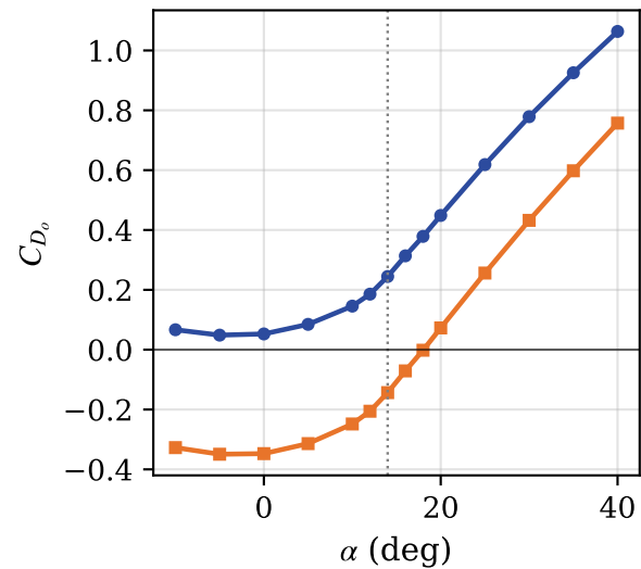
(d) Net axial force
