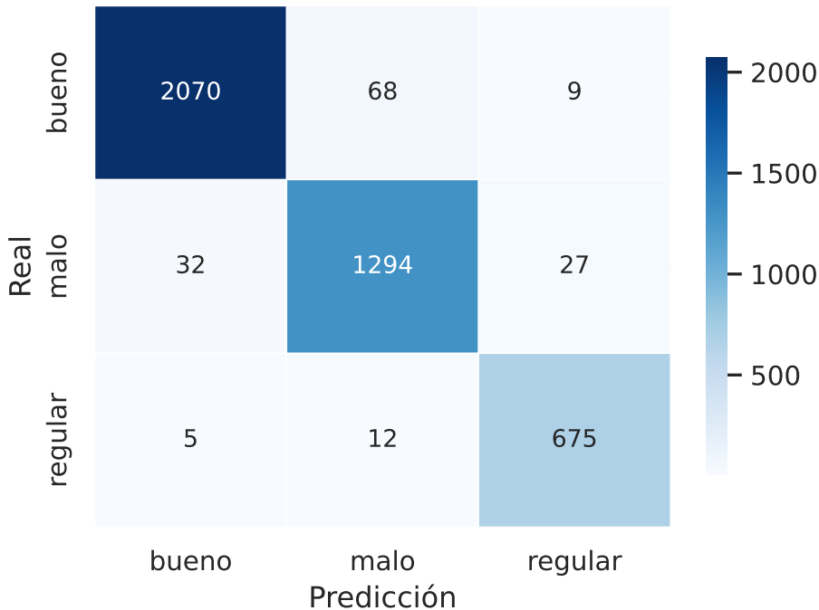
Matriz de confusión — Random Forest
