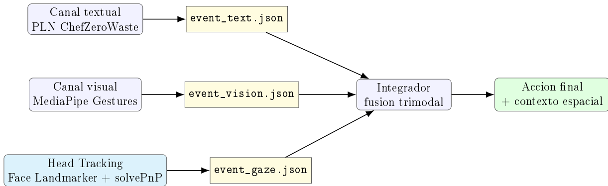
Figura 15: Arquitectura con tres canales: texto, gestos y head tracking.
