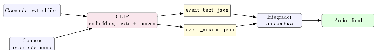
Figura 8: Arquitectura de la ampliacion zero-shot con CLIP.
