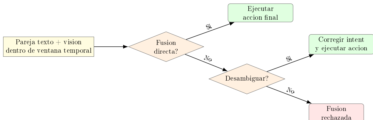
Figura 13: Flujo de decision del integrador con desambiguacion mutua.
