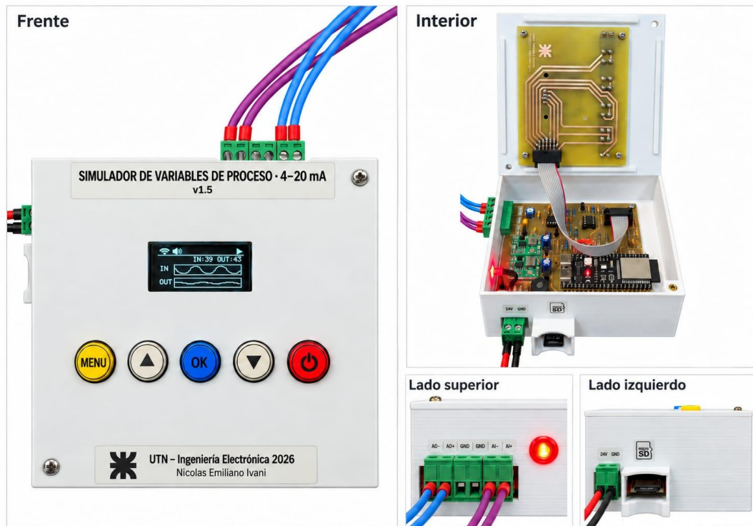
Figura 4.13 – Montaje final del hardware del simulador
