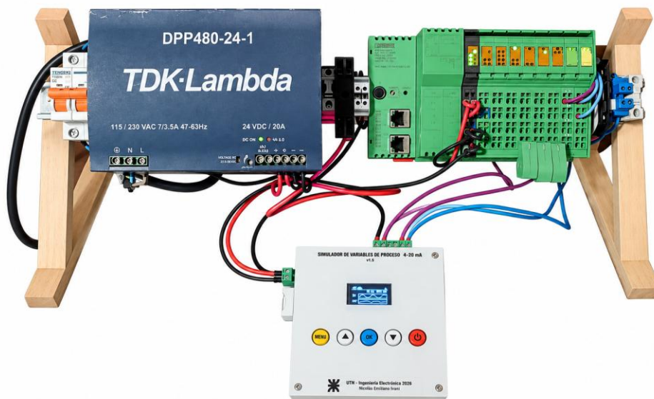
Figura 4.14 – Montaje final del banco de pruebas del PLC con el simulador
