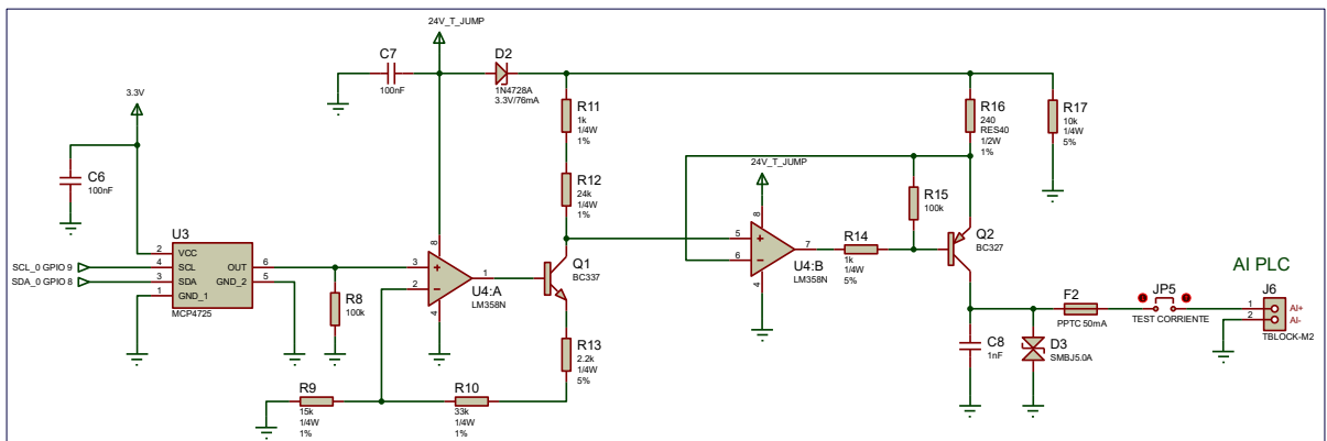
Conversor digital-analógico
