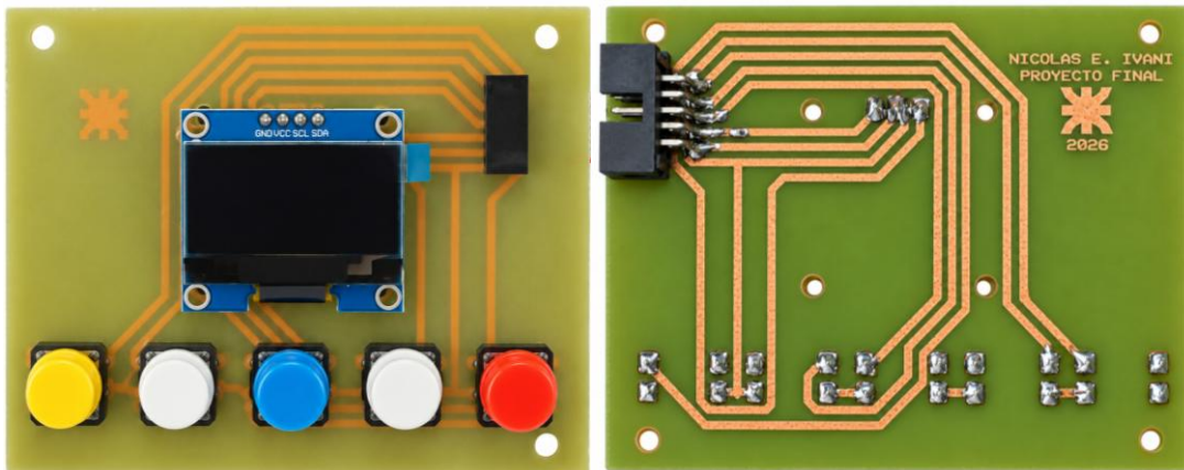
Figura 4.13 – Placa interfaz de usuario fabricada vista superior e vista inferior
