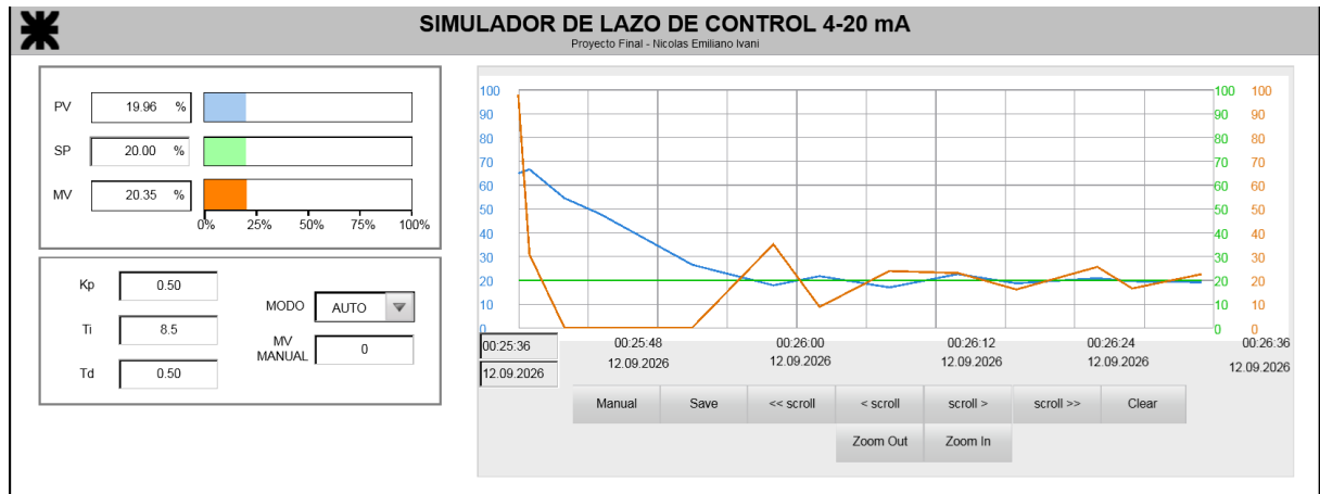
Figura 6.4 – Pantalla de operación del lazo en WebVisit
