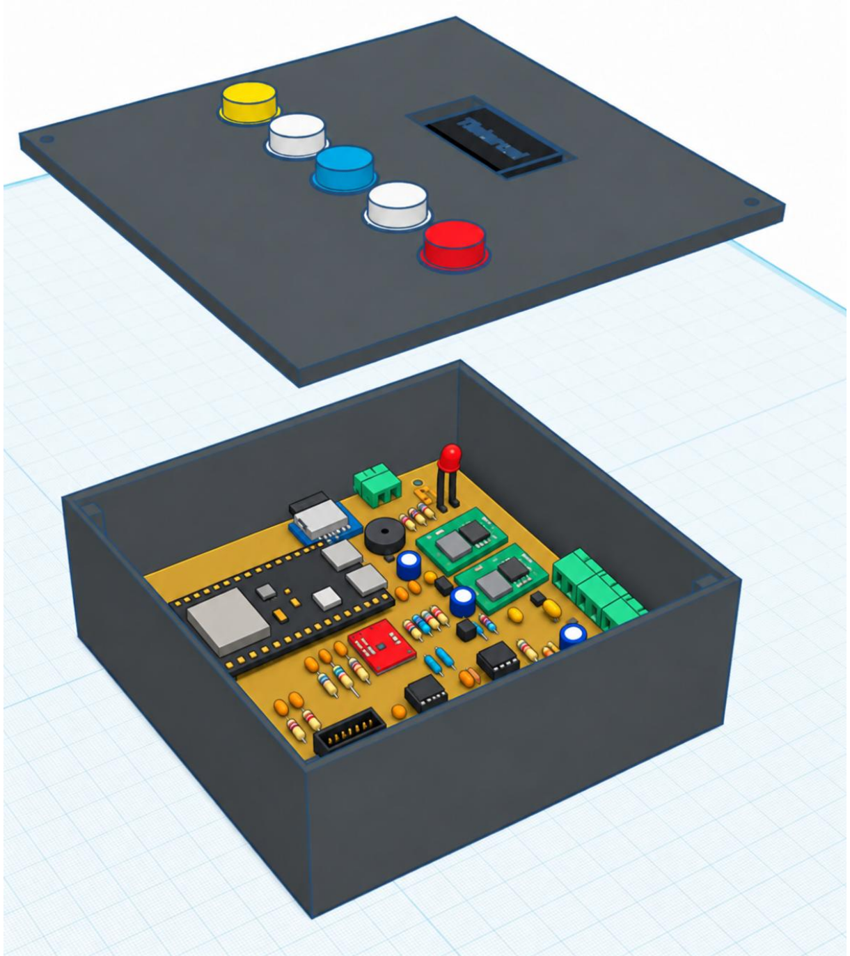
Figura 4.12 – Modelo 3D del gabinete del simulador
