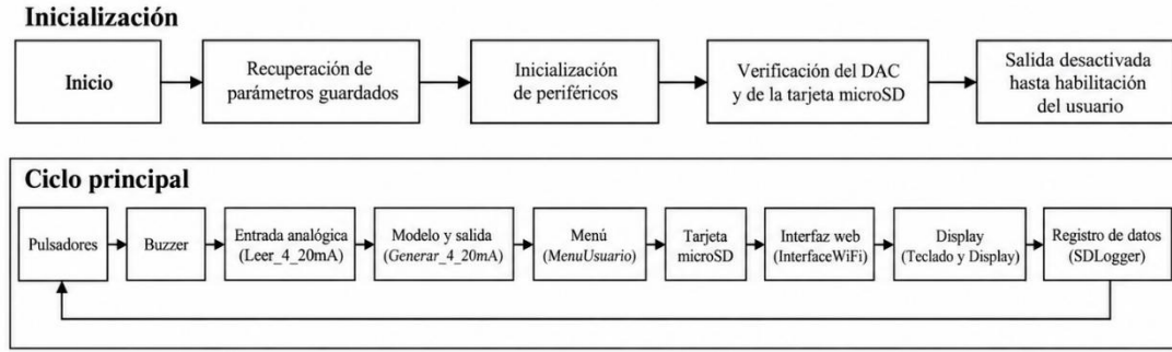
Figura 5.1 – Organización general del firmware
