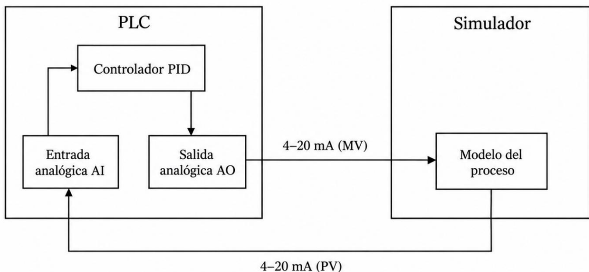
Figura 3.1 – Conexión general entre el PLC y el simulador
