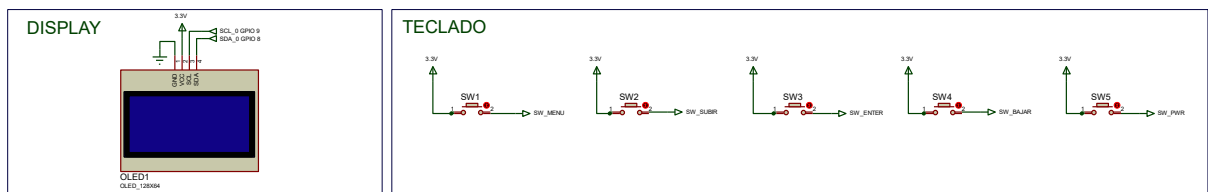
Figura 4.5 – Circuitos de la interfaz local en la placa superior
