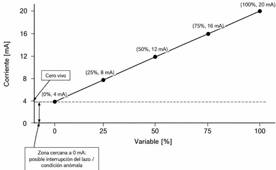
Figura 2.1 – Representación de una variable mediante una señal 4–20 mA
