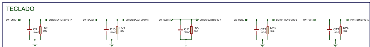
Figura 4.6 – Circuitos asociados a la interfaz local en la placa base
