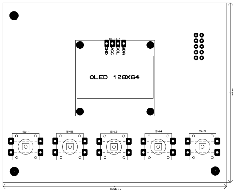
Figura 4.11 – Diseño PCB vista superior de la placa interfaz de usuario
