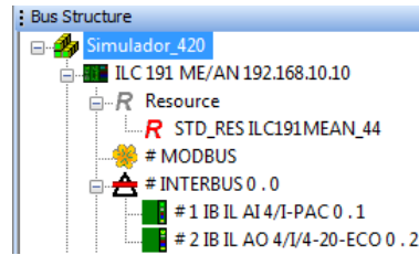
Figura 6.1 – Configuración del PLC y del módulo de entrada analógica
