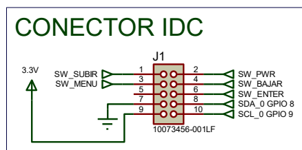
Figura 4.7 – Interconexión entre la placa base y la placa de interfaz
