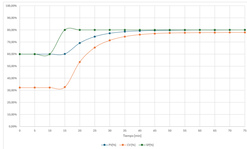
Figura 3.3 – Ejemplo de respuesta histórica de un lazo de control industrial
