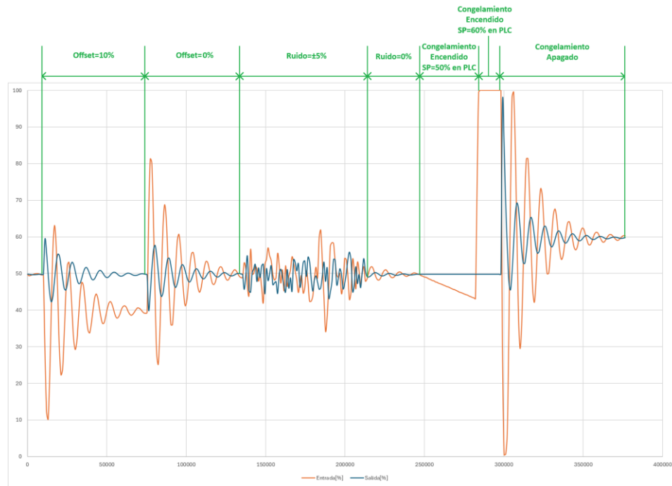
Figura 7.5 – Respuesta del lazo ante offset, ruido de medición y congelamiento
