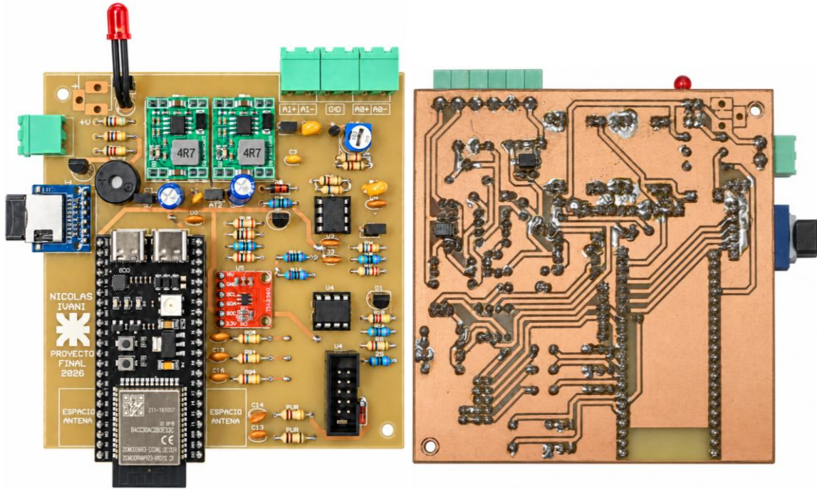
Figura 4.10 – Placa base fabricada vista superior e vista inferior
