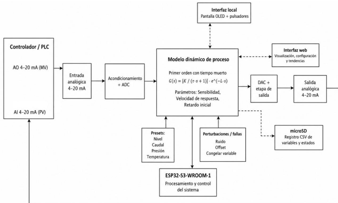
Figura 1.2 – Arquitectura general del simulador de variables de proceso
