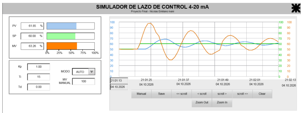
Figura 6.4 – Pantalla de operación del lazo en WebVisit
