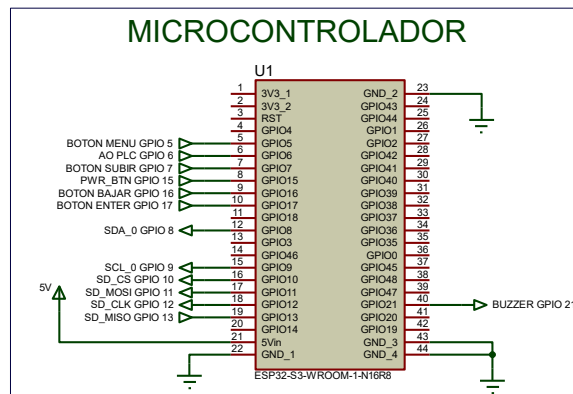
Figura 4.2 – Conexiones principales del ESP32-S3
