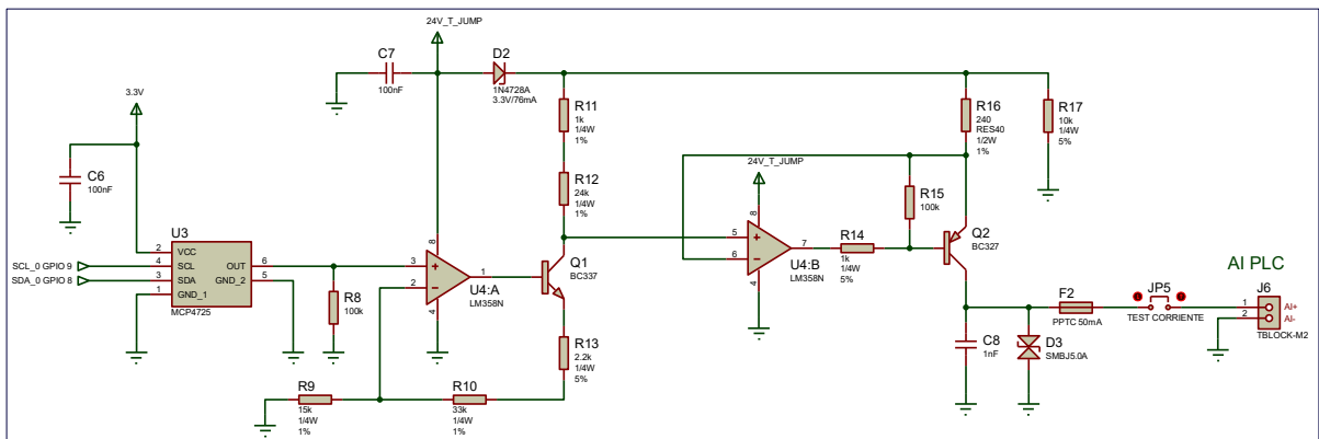
Figura 4.4 – Circuito de salida de 4–20 mA
