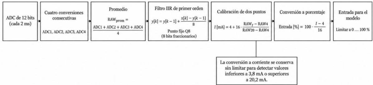
Figura 5.2 – Procesamiento digital de la entrada
