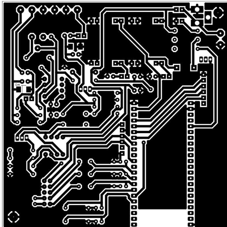
Figura 4.9 – Diseño PCB vista inferior de la placa base
