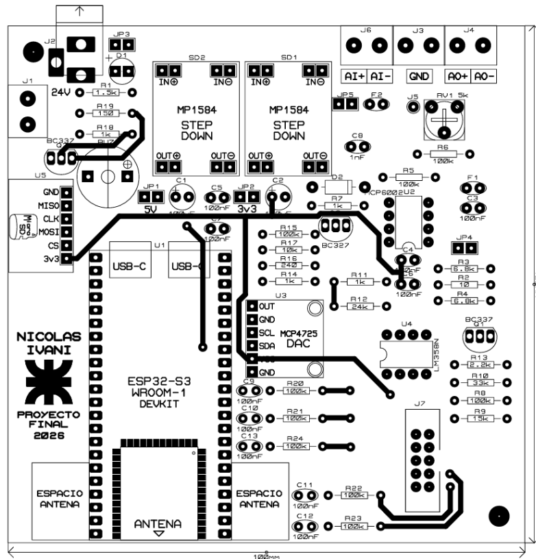
Figura 4.8 – Diseño PCB vista superior de la placa base
