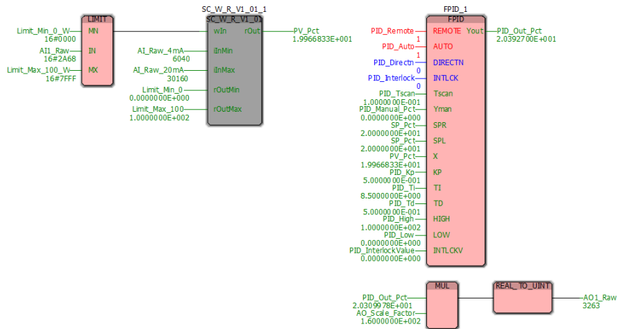
Figura 6.3 – Implementación del controlador FPID en PC Worx
