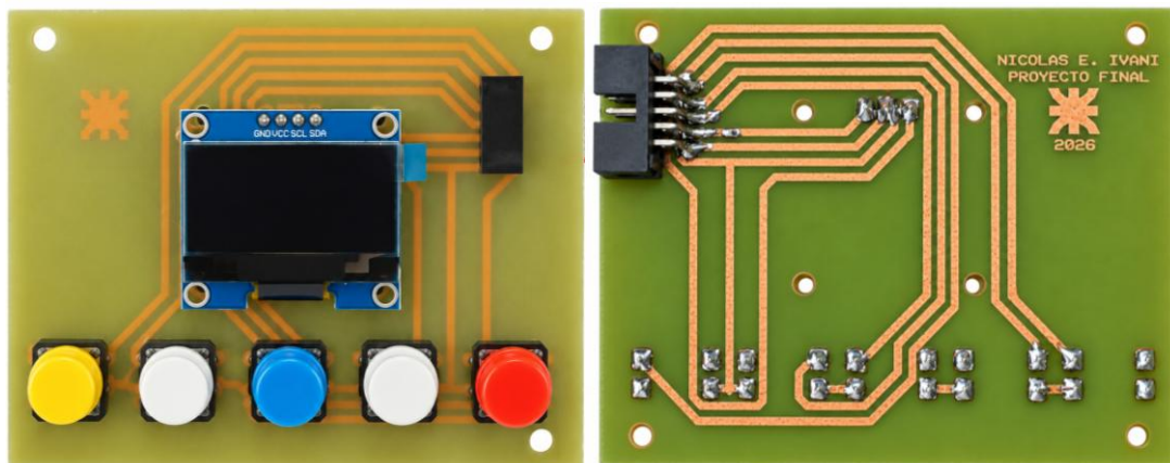
Figura 4.13 – Placa interfaz de usuario fabricada vista superior e vista inferior
