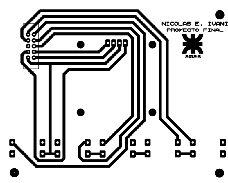
Figura 4.12 – Diseño PCB vista inferior de la placa interfaz de usuario
