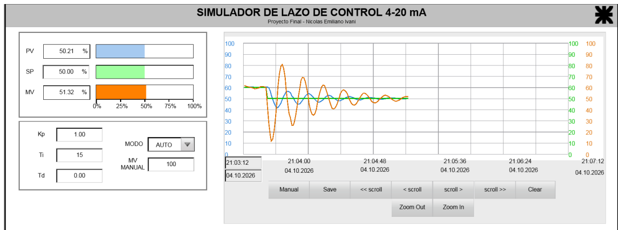
Figura 7.1 – Respuesta del lazo de control con el PLC.
