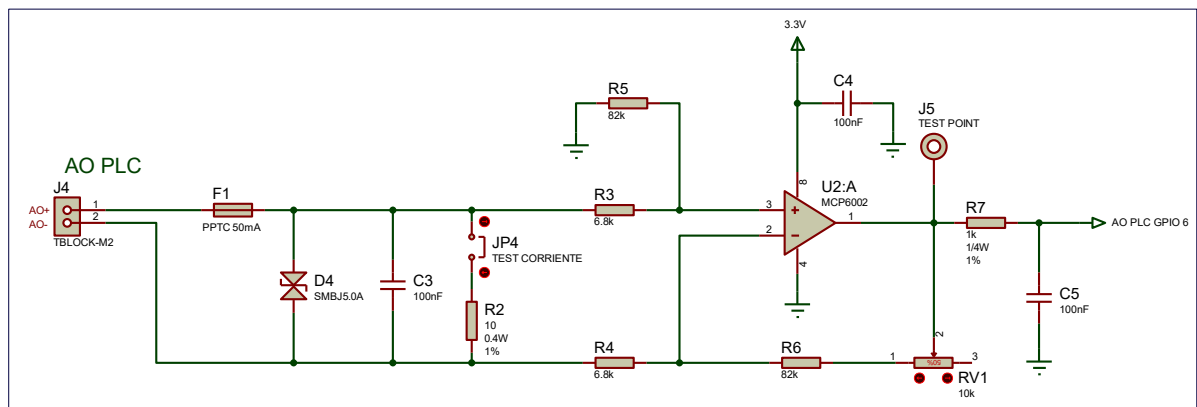
Figura 4.3 – Circuito de entrada de 4–20 mA
