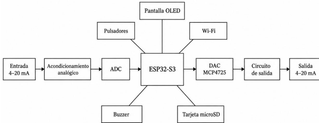
Figura 3.2 – Arquitectura interna del simulador
