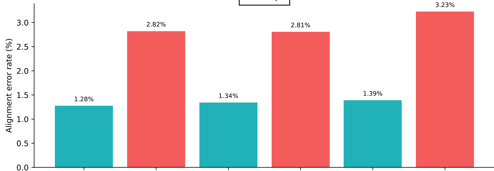
minimap2
