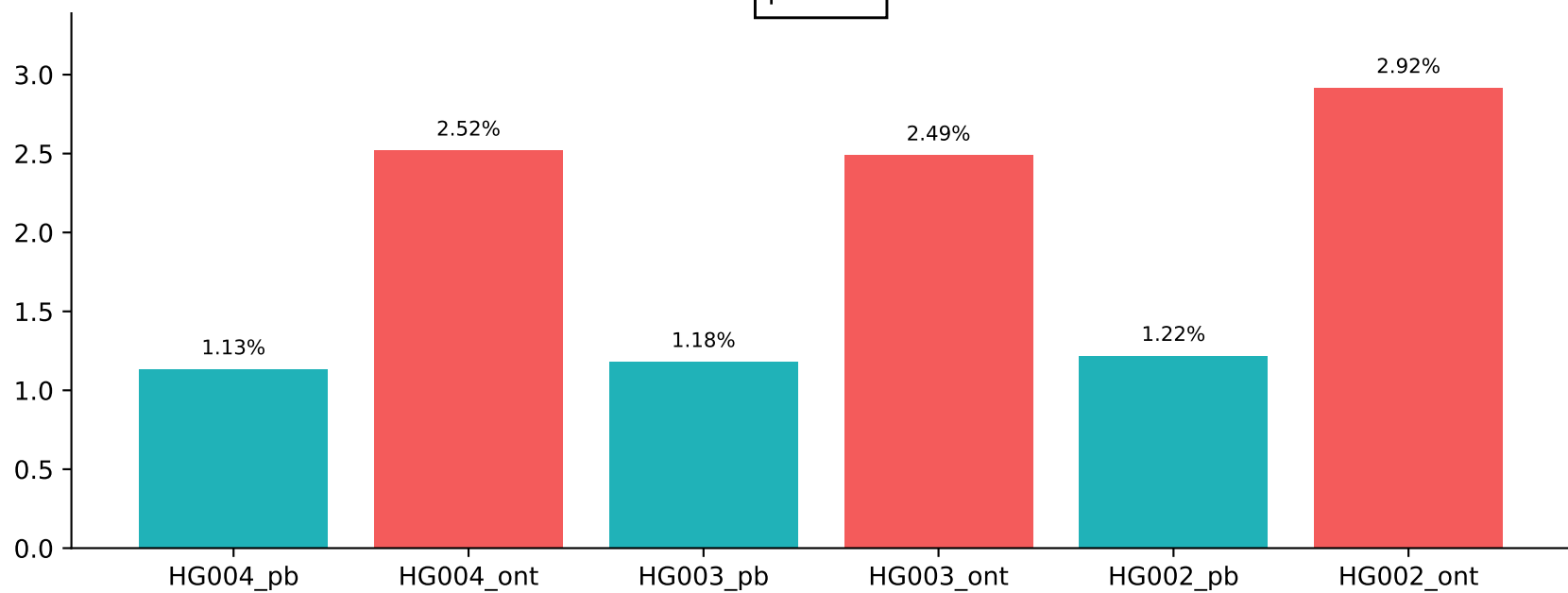
pbmm2
