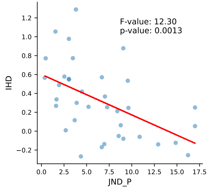
JND_P vs IHD
