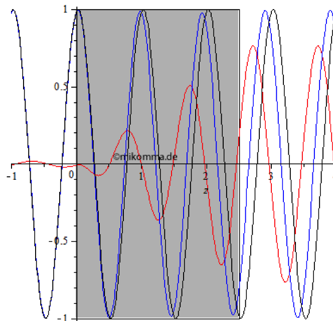
Abbildung 2.1: Visualisierung der Wellenlängenverkürzung im Medium durch die Phasenverzögerung der gestreuten Wellen. Die Primärwelle (von links einfallend) ist schwarz, das Gesamtfeld der gestreuten Dipolwellen rot und die resultierende transmittierte und reflektierte Welle blau dargestellt.[2]
