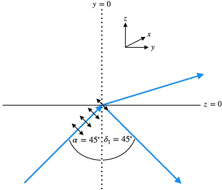
Abbildung 4.4: Übergang einer Elektromagnetischen Welle ins optisch dünnere Medium bei einem Einfallswinkel von 45^\circ .
