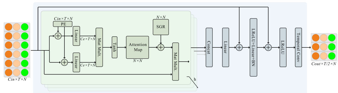
Figura 4.4: Esquema del módulo de atención de keypoints del cuerpo. Imagen de [9]
