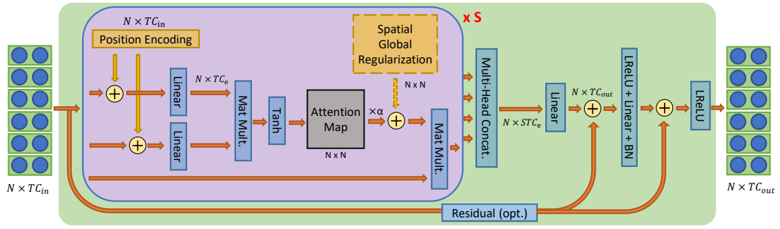
Figura 3.7: Esquema del módulo de atención espacial. Obtenido de [12]
