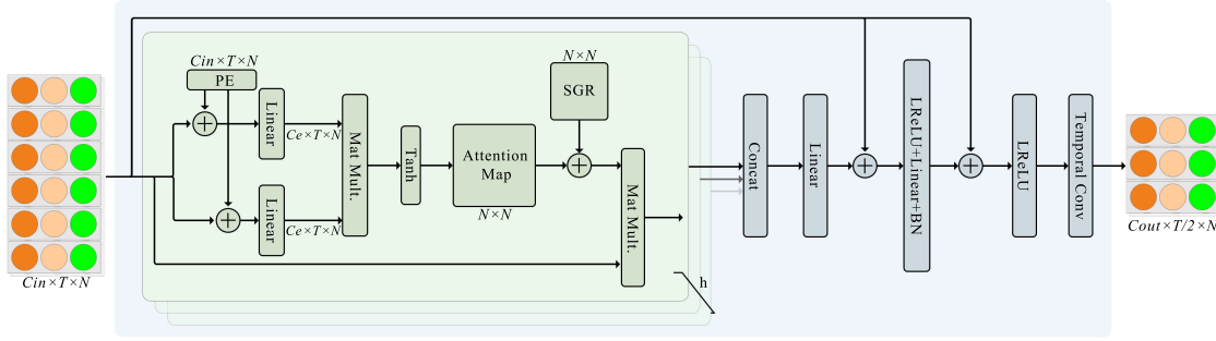
Figura 4.4: Esquema del módulo de atención de keypoints del cuerpo. Imagen de [9]
