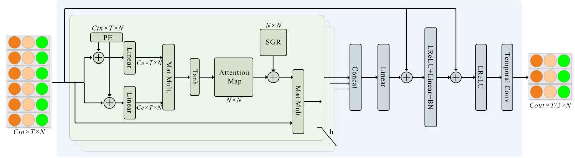
Figura 4.3: Esquema del módulo de atención de keypoints . Imagen de [9]
