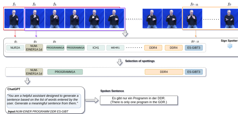
Figura 2.3: Estructura del modelo Spotter+GPT propuesto por Sincan et al. [21]
