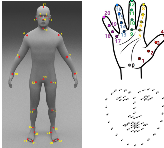
Figura 4.2: Distribución de keypoints anatómicos en el formato Halpe-136 [7].
