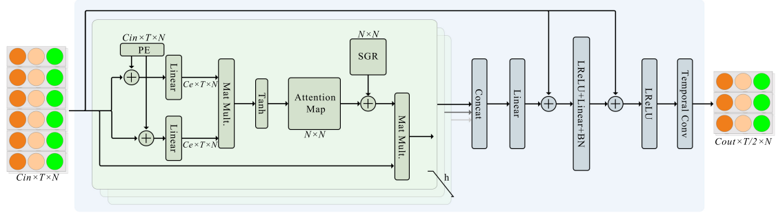
Figura 4.5: Esquema del módulo de atención de keypoints del cuerpo. Se toma h = 6 . Imagen de [20]
