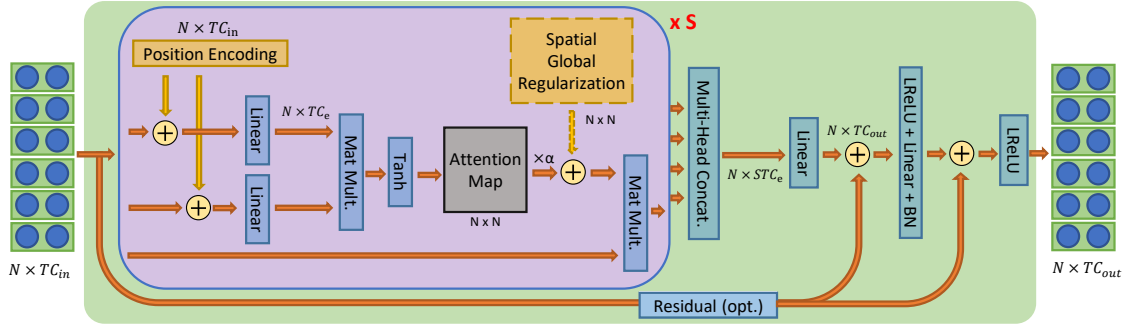
Figura 3.6: Esquema del módulo de atención espacial . Obtenido de [23]
