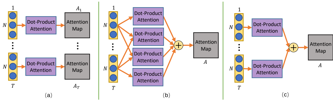
Figura 3.2: Las tres estrategias propuestas en [23]. Gráfico sacado de ese papel.
