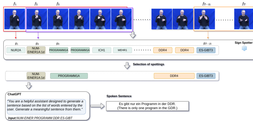
Figura 2.3: Estructura del modelo Spotter+GPT propuesto por Sincan et al. [22]
