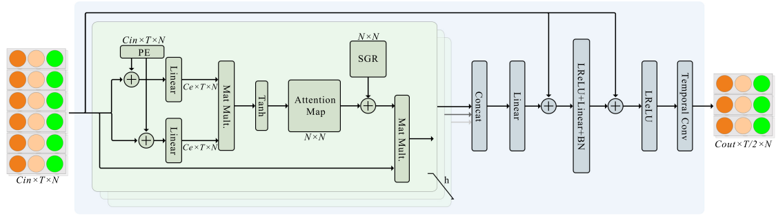
Figura 4.5: Esquema del módulo de atención de keypoints del cuerpo. Se toma h = 6 . Imagen de [21]
