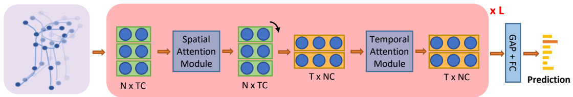
Figura 3.7: Esquema de la red. Obtenido de [27]
