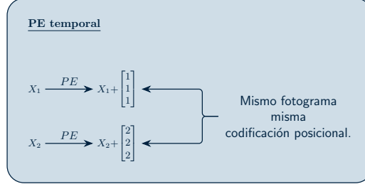
Figura 3.5: Consideramos 2 fotogramas con 3 puntos clave cada uno. Esto es un esquema de lo que ocurre.
